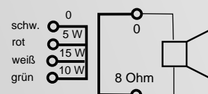
Anschlussbild SPH-15
